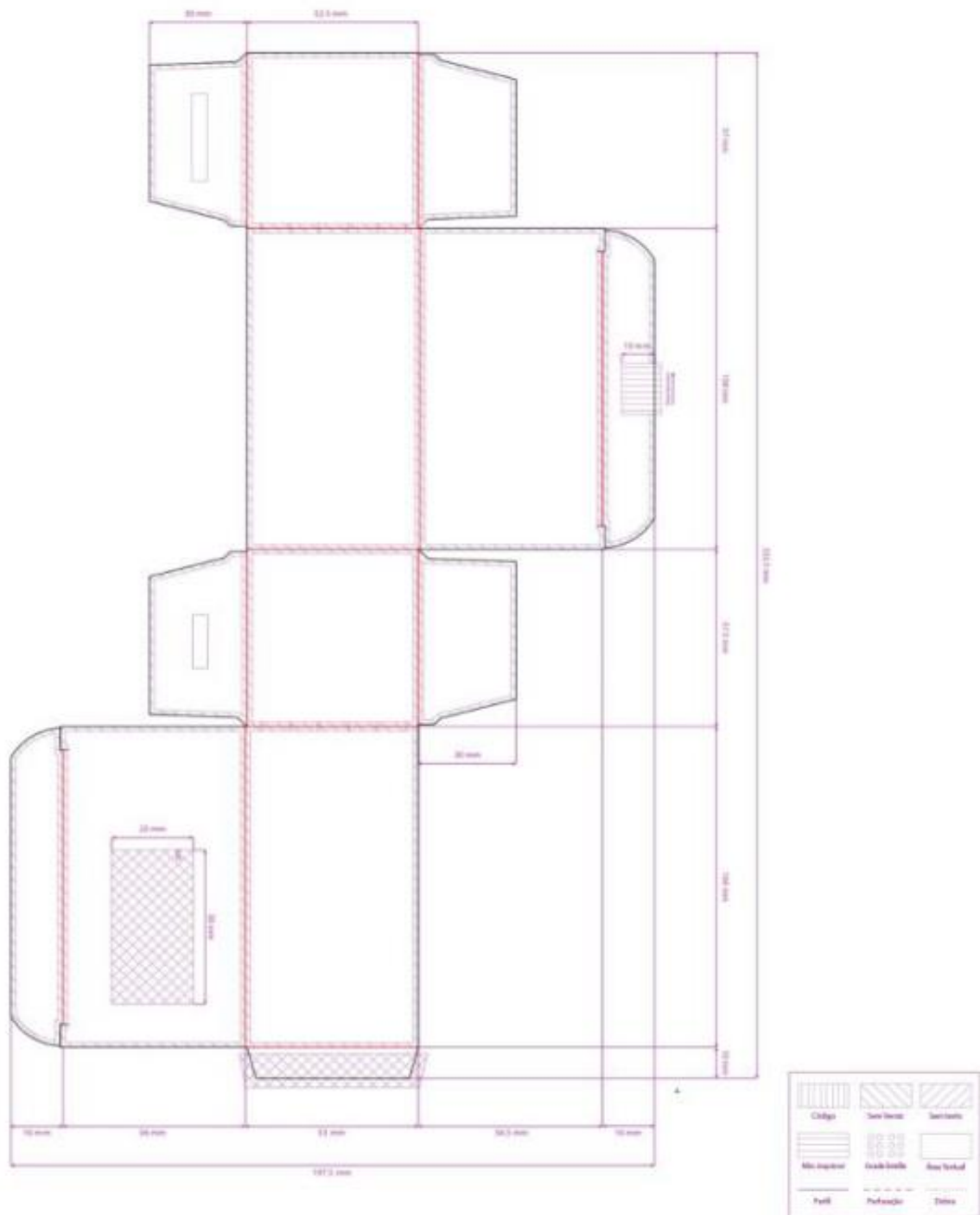
Figura 6 - Desenho técnico com dimensões do cartucho.
