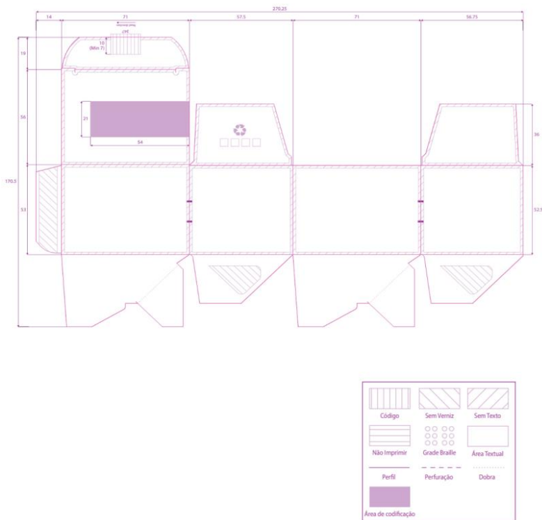
Figura 2 – Desenho técnico com dimensões do cartucho
