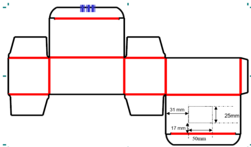
Figura 5 – Área de reserva de verniz (zona de impressão sem verniz).
