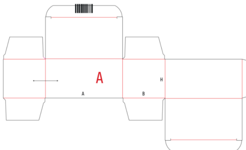
Figura 4 – Formato do cartucho e posição do PharmacoDE. Seta indicando direção das fibras e letra A indicando direção de impressão.
